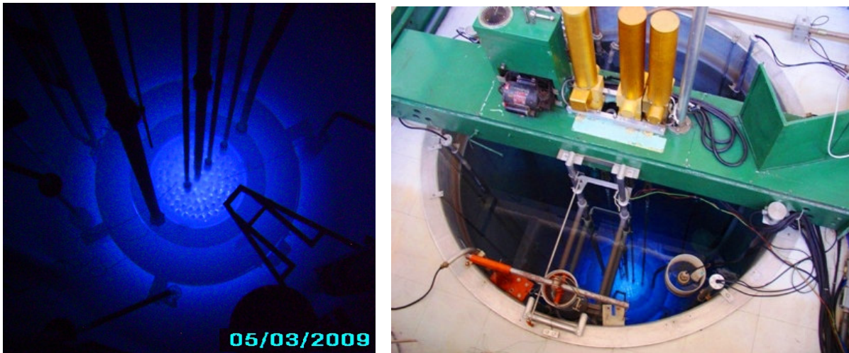
Figura 2. Reator nuclear TRIGA IPR-R1, vista do núcleo e poço com o reator crítico
