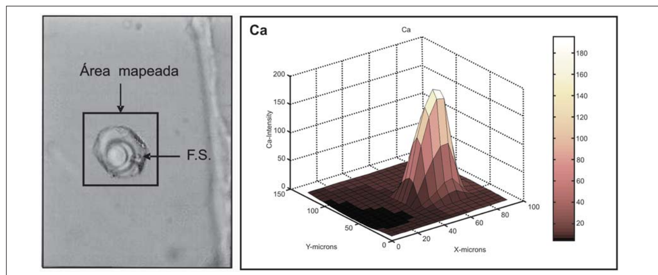
Figura 2 - A fotomicrografia mostra uma inclusão fluida polifásica em esmeralda do garimpo de Capoeirana, Nova Era, MG. O tamanho da inclusão fluida é de 50 \mu m, estando localizada a 14 \mu m de profundidade em relação à superfície da lâmina. A imagem ao lado da fotomicrografia mostra uma representação gráfica da presença de cálcio numa das fases sólidas (F. S.) presentes na inclusão fluida.
