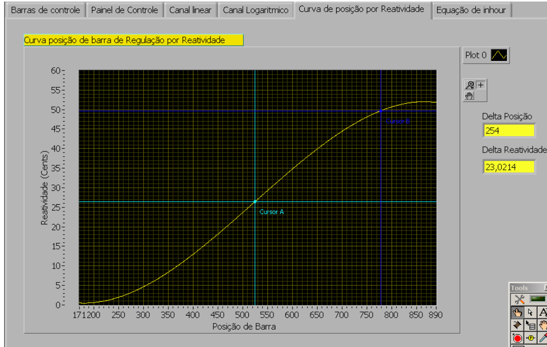
Fig. 4. Reatividade em função da posição da Barra de Regulação.
