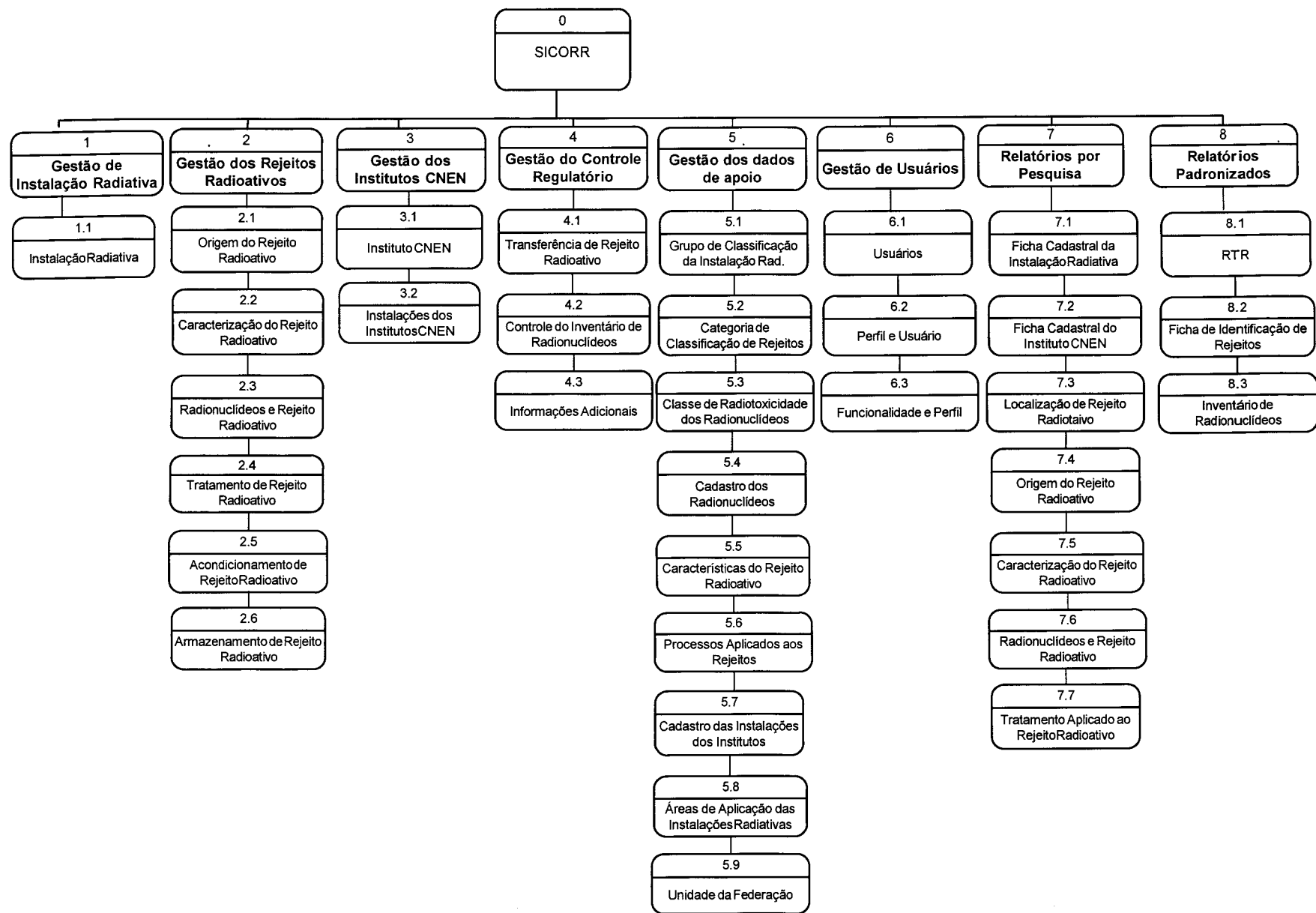
FIGURA 6 - Diagrama Hierárquico Funcional do SICORR
