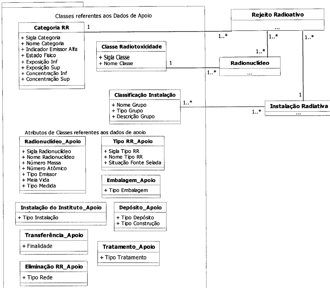
FIGURA 9 - Classes e atributos referentes aos dados de apoio
