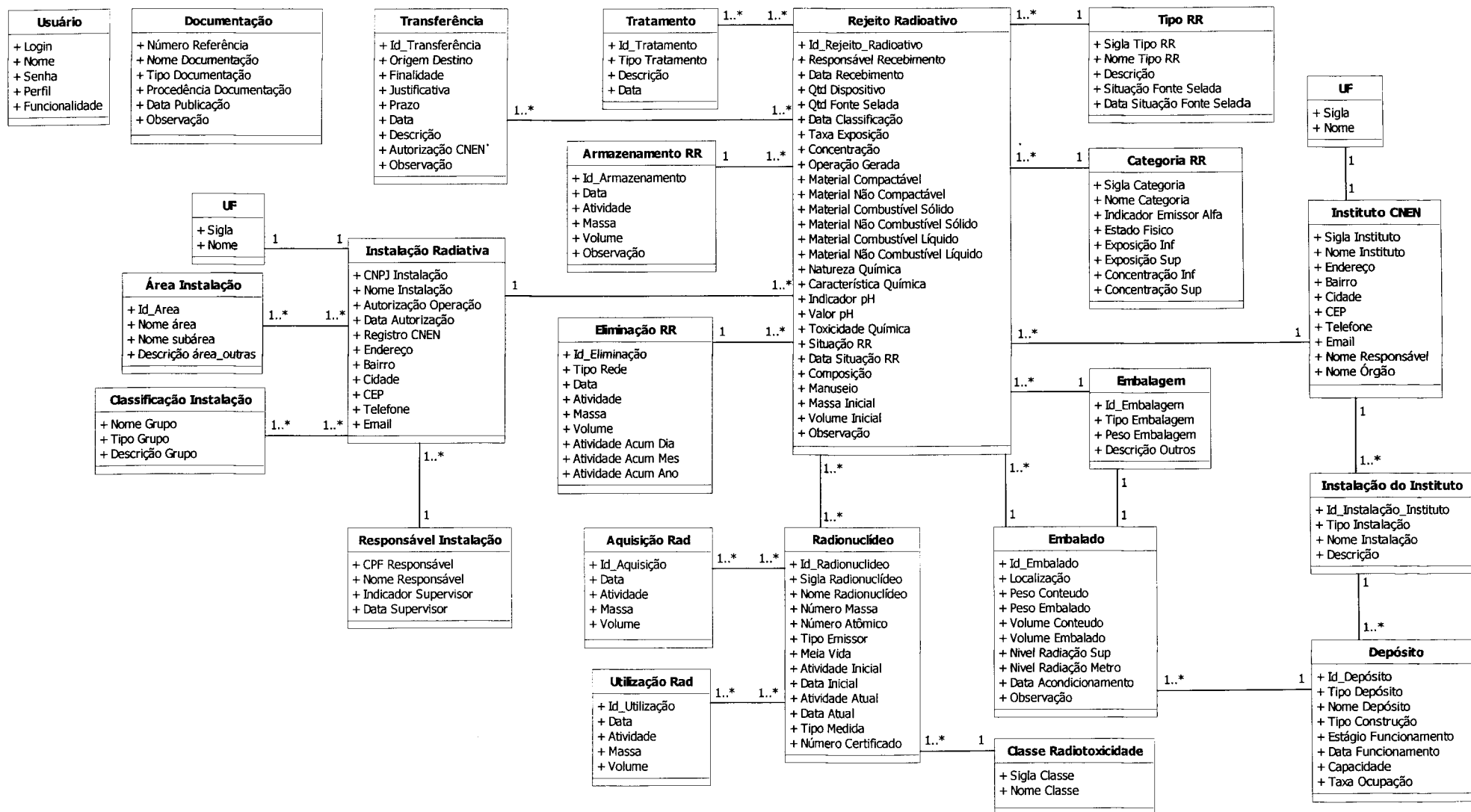
FIGURA 8 - Diagrama de classes persistentes do SICORR
