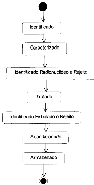
FIGURA 4 - Diagrama de Estado - Gestão de rejeitos radioativos
