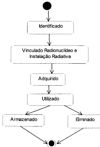
FIGURA 5 - Diagrama de Estado - Controle de inventário de radionuclídeos
