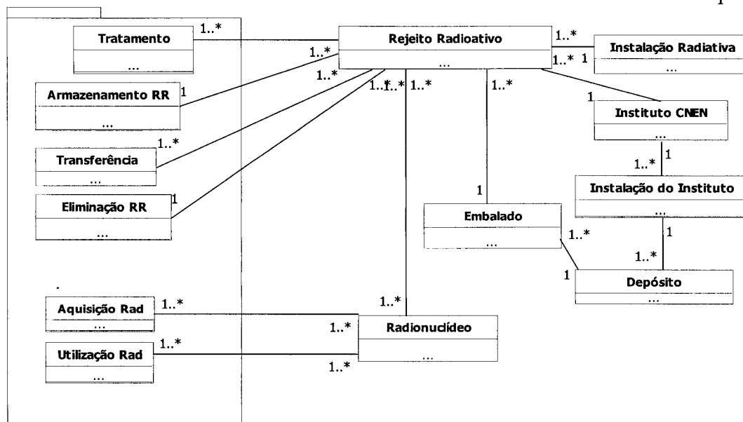
FIGURA 10 - Classes referentes aos processamentos de rejeito radioativo e de radionuclídeo
