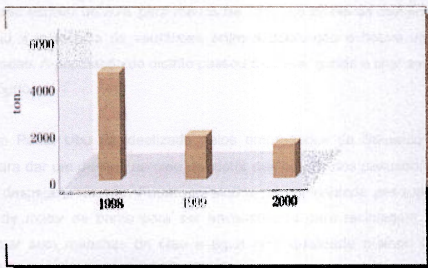
Figura 12: Emissão de partículas para a atmosfera
