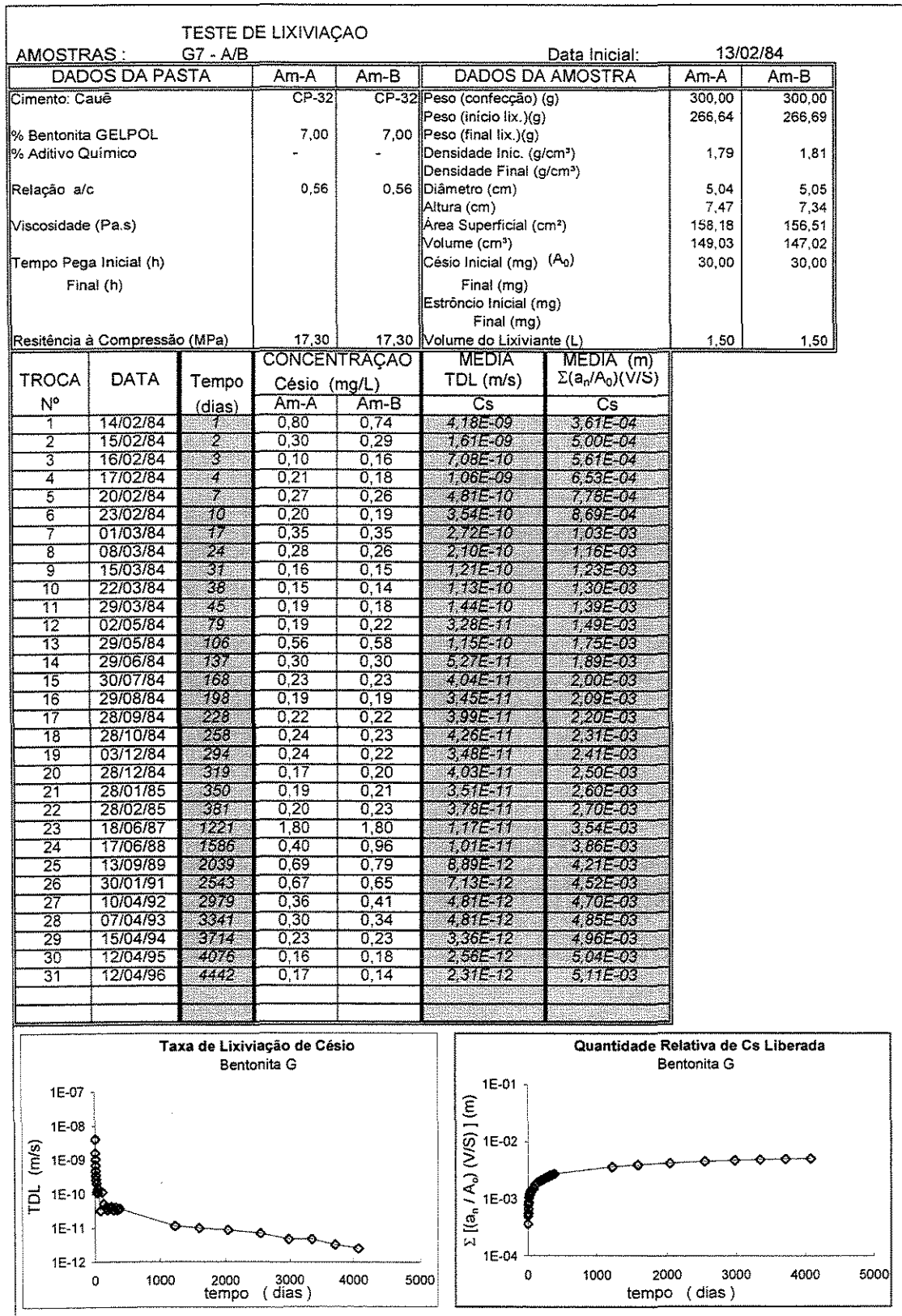
FIGURA 4.6 Protocolo para acompanhamento do ensaio de lixiviação
