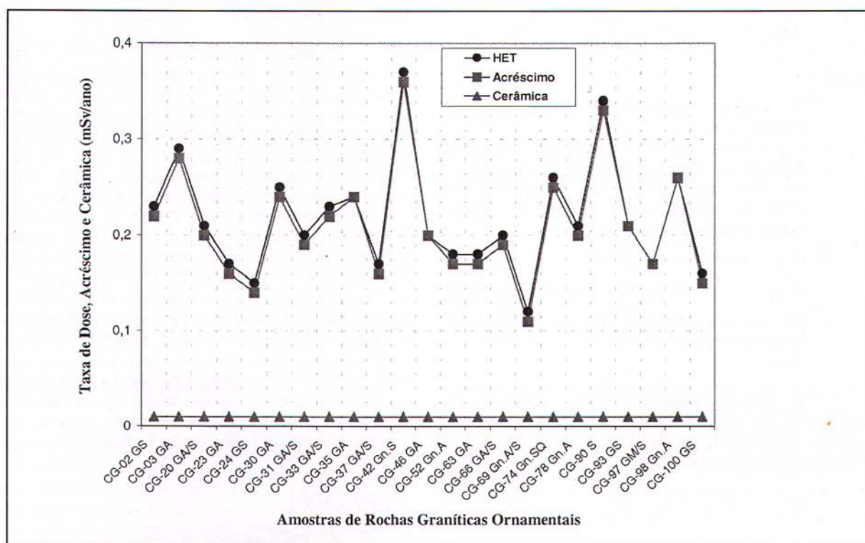
Figura 2- Taxa de dose, acréscimo utilizando-se rochas graníticas com elementos radioativos totais ( U_3O_8 e ThO_2 ) acima de 60 ppm (GA - granito alcalino, Gn.A - gnaiss alcalino, GA/S - granito alcalino/sienítico, Gn.A/S - gnaiss alcalino/sienítico, GS - granito sienítico, Gn.S - gnaiss sienítico, GM - granito monzonítico, S - sienito e Gn.SQ - gnaiss sienito quartzoso) em lugar do material cerâmico
