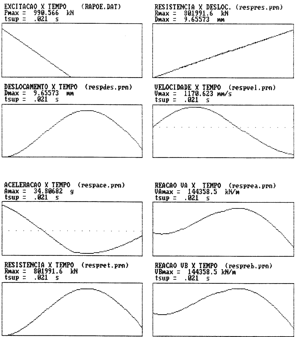
Figura 30 - Resultados gráficos do programa RESPOD para o arquivo de dados RAPOE.DAT (laje em apoio simples com deslocamento máximo na faixa elástica )
